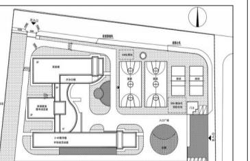
附件二:福州市台江第二实验小学项目拟调整总平面
