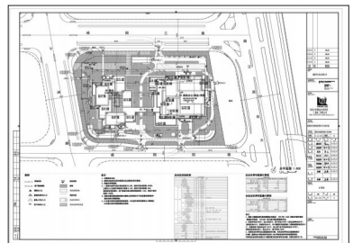
拟调整总平面
