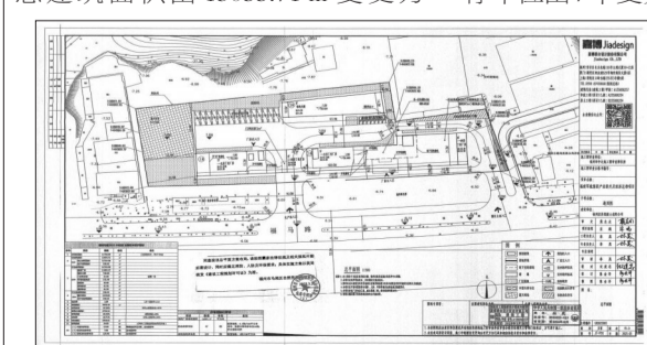
项目原总平面规划方案
