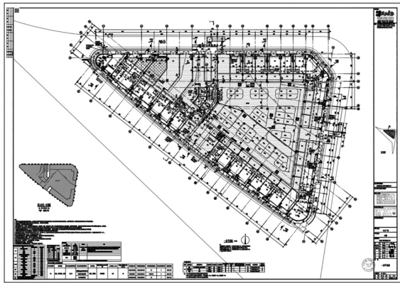
一层平面图修改前
