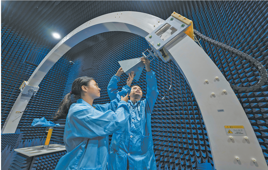
闽都创新实验室内，科研人员开展电磁兼容材料测量实验。本报记者 林双伟摄
