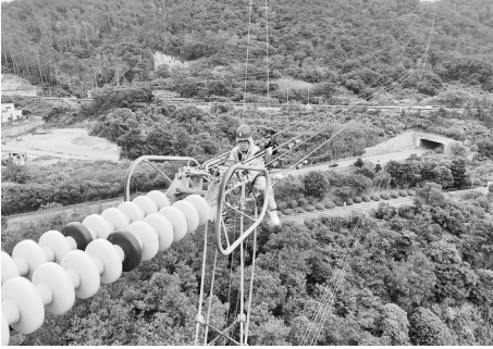
身穿屏蔽服的等电位作业人员在50多米高空作业。(国网福州供电公司供图)
